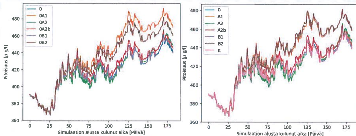
Kuva 18: Kokonaistyyppipitoisuus ( \mu\text{g l}^{-1} ) Sunisenselän vedenottopaikalla 2.5.2010–31.10.2010. Vasemmalla ne vaihtoehdot, joissa ei ole Kutilan kanavaa, ja oikealla ne, joissa on Kutilan kanava.
