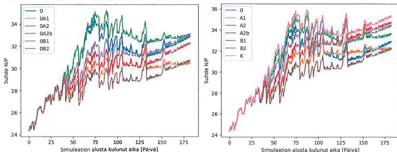
Kuva 26: Ravinnesuhde, N/P-luku, Niemisenselällä aikavälillä 2.5.2010–31.10.2010 eri vaihtoehtoilla.
