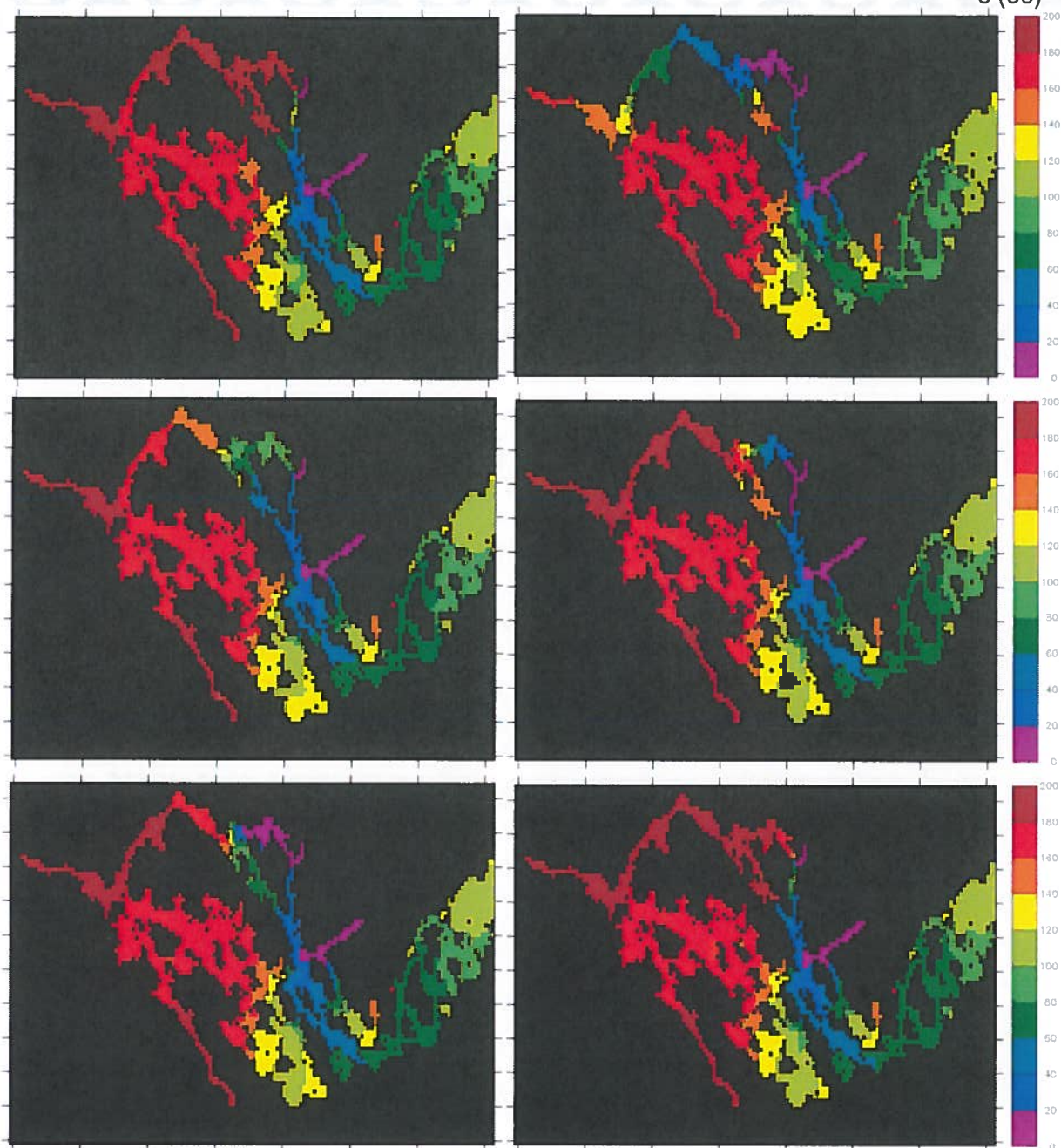
Kuva 6: Veden ikä 182 päivää tarkastelujakson alusta vaihtoehtoissa, joissa Kutilan kanava on rakennettu. Ylhäällä vasemmalla vaihtoehto A1 ja oikealla A2. Keskellä vasemmalla vaihtoehto B1 ja oikealla B2. Alhaalla vasemmalla vaihtoehto A2b ja oikealla vaihtoehto K, eli pelkkä Kutilan kanava.
