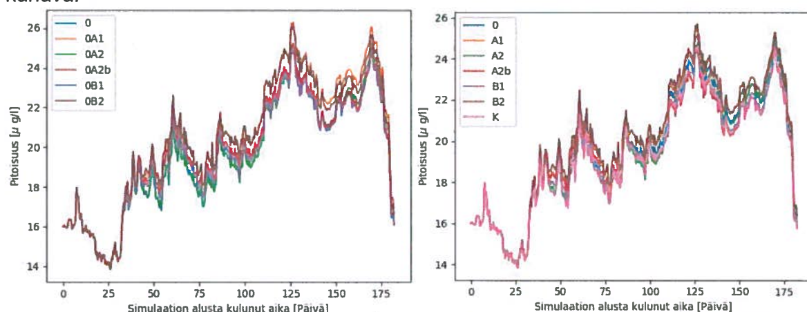
Kuva 17: Kokonaisfosforipitoisuus ( \mu\text{g/l}^1 ) Sunisenselän vedenottopaikalla 2.5.2010–31.10.2010. Vasemmalla ne vaihtoehdot, joissa ei ole Kutilan kanavaa, ja oikealla ne, joissa on Kutilan kanava.
