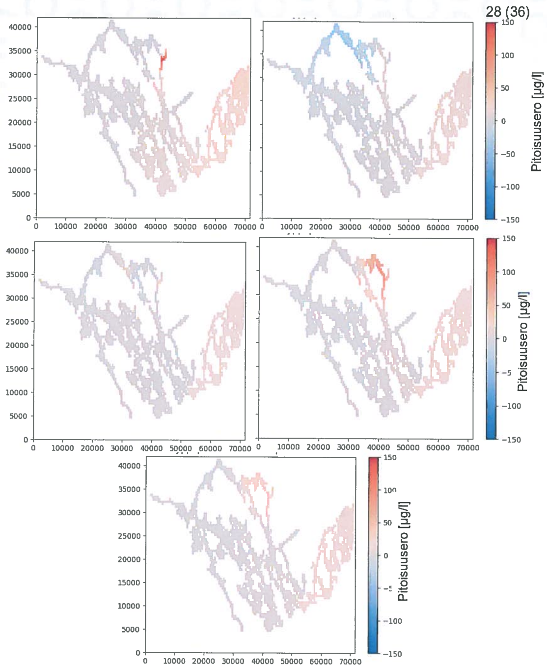
Kuva 35: Kutilan kanavan vaikutus typpipitoisuuksiin tarkastelujakson lopussa eri pumppaamovaihtoehtoissa. Ylhäällä vasemmalla on verrattu vaihtoehtoja 0A1 ja A1 sekä vasemmalla vaihtoehtoja 0A2 ja A2. Keskellä vasemmalla on verrattu vaihtoehtoja 0B1 ja B1 sekä oikealla 0B2 ja B2. Alhaalla on verrattu vaihtoehtoja 0A2b ja A2b. Punainen sävy tarkoittaa Kutilan kanavan rakentamisen vähentäneen pitoisuuksia.
