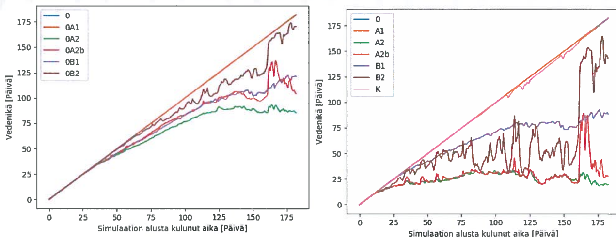
L1: Veden ikä Maaveden havaintopisteessä eri vaihtoehtoissa. Vasemmalla vaihtoehdot, joissa Kutilan kanavaa ei ole ja oikealla ne, joissa se on.
