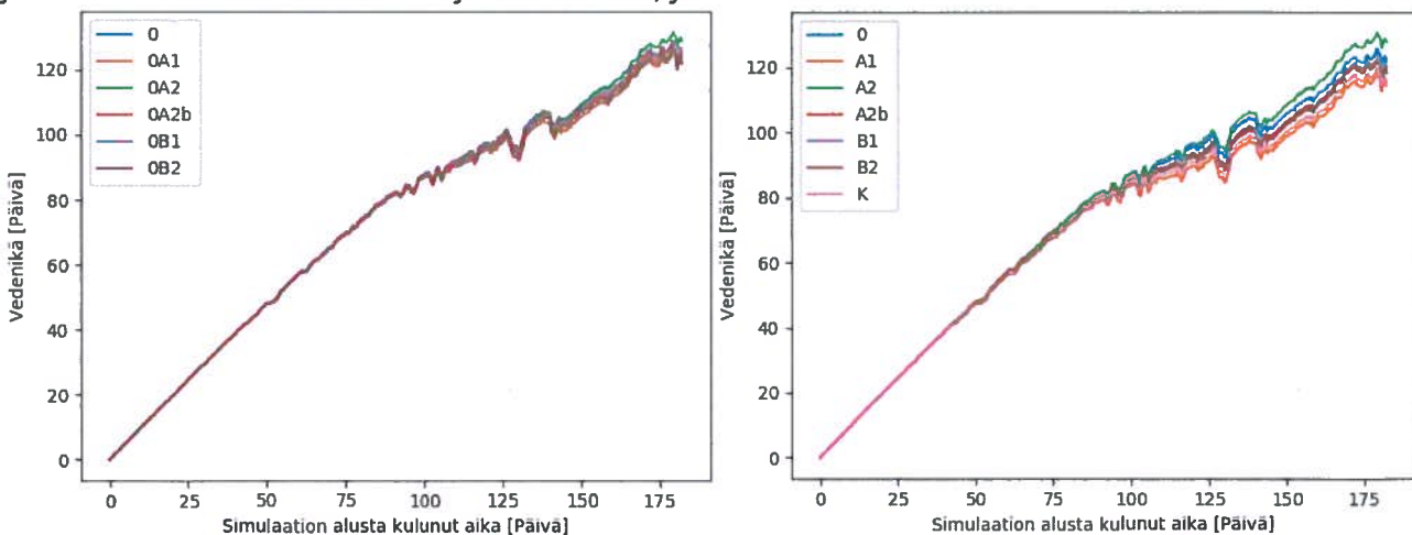
L3: Veden ikä Sunisenselän havaintopisteessä eri vaihtoehtoissa. Vasemmalla vaihtoehdot, joissa Kutilan kanavaan ei ole ja oikealla ne, joissa se on.
