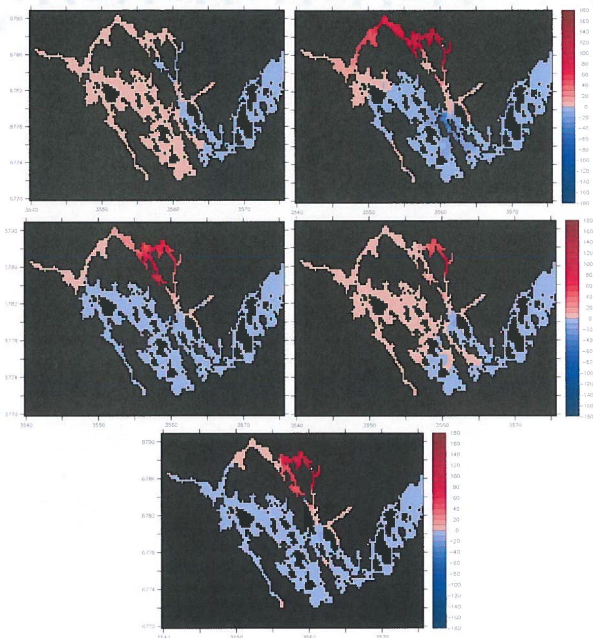
L6: Veden ikä muuttujan erotus nykytilasta (0) ajanhetkellä 182 päivää simulaation alusta. Ylärivillä vasemmalla erotus 0- 0A1, oikealla erotus 0-0A2. Keskellä vastaavasti vasemmalla erotus 0-0B1 ja oikealla erotus 0-0B2. Alarivillä erotus 0-0A2b. Punainen väri tarkoittaa että veden ikä on nykytilassa vanhempaa ja uusi vaihtoehto nuorentaa sitä.
