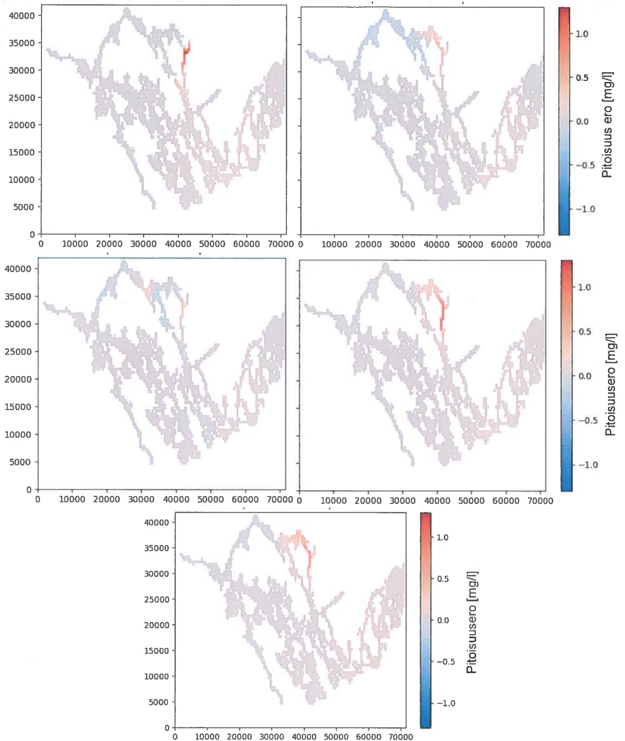
Kuva 33: Kutilan kanavan vaikutus kiintoainepitoisuuseroihin tarkastelujakson lopussa verrattaessa eri pumppaamovaihtoehtoja. Ylhäällä vasemmalla on verrattu vaihtoehtoja 0A1 ja A1 sekä oikealla vaihtoehtoja 0A2 ja A2. Keskellä vasemmalla on verrattu vaihtoehtoja 0B1 ja B1 sekä oikealla 0B2 ja B2. Alhaalla on verrattu vaihtoehtoja 0A2b ja A2b. Punainen sävy kertoo Kutilan kanavan rakentamisen vähentäneen pitoisuuksia.
