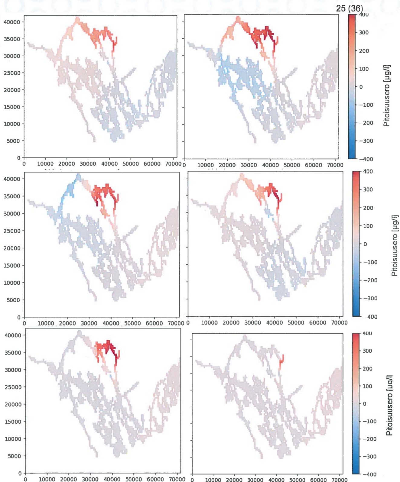
Kuva 32: Kokonaistyyppipitoisuuden erot pintakerroksessa verrattaessa nykytilaa vaihtoehtoihin, joissa Kutilan kanava on. Ylhäällä vasemmalla on vaihtoehtojen erotus 0-A1 ja oikealla 0-A2. Keskellä vasemmalla on vaihtoehtojen erotus 0-B1 ja oikealla 0-B2. Alhaalla vasemmalla on vaihtoehtojen erotus 0-A2b ja oikealla 0-K. Punainen värisävy tarkoittaa suurempaa pitoisuutta nykytilassa kuin vaihtoehdossa.
