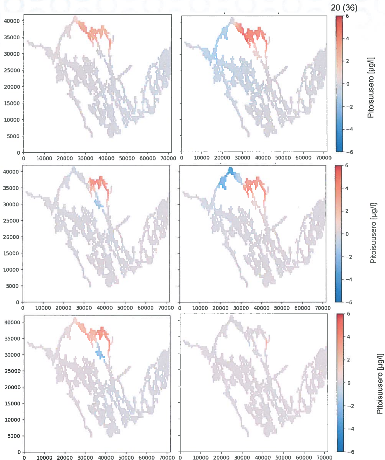
Kuva 28: Kiintoainepitoisuuden erot pintakerroksessa verrattaessa nykytilaa (0) vaihtoehtoihin, joissa on Kutilan kanava. Ylhäällä vasemmalla on vaihtoehtojen erotus 0-A1 ja oikealla erotus 0-A2. Keskellä vasemmalla on vaihtoehtojen erotus 0-B1 ja oikealla erotus 0-B2. Alhaalla vasemmalla on vaihtoehtojen erotus 0-A2b ja oikealla erotus 0-K. Punainen värisävy tarkoittaa suurempaa pitoisuutta nykytilassa kuin vaihtoehdossa.
