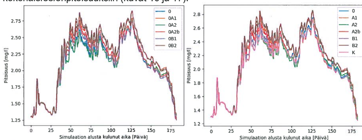
Kuva 16: Kiintoainepitoisuus ( \text{mg/l}^1 ) Sunisenselän vedenottopaikalla 2.5.2010–31.10.2010. Vasemmalla ne vaihtoehdot, joissa ei ole Kutilan kanavaa, ja oikealla ne, joissa on Kutilan kanava.
