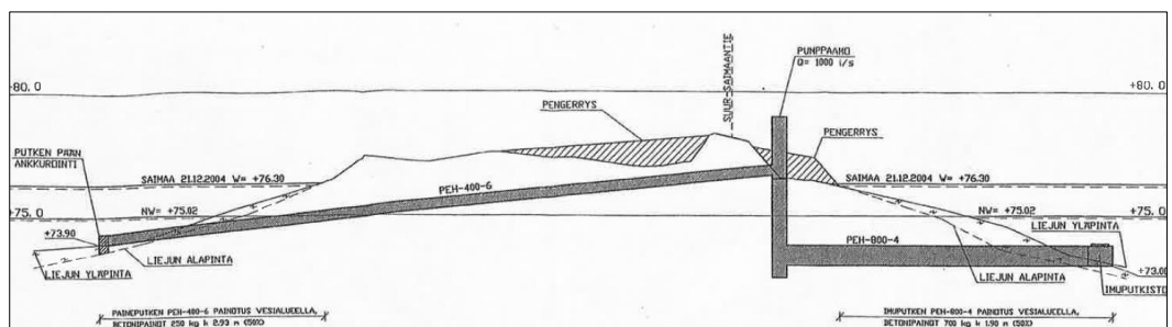
Kuva 10. Ote pienen pumppaamon yleissuunnitelman pituusleikkauksesta (Insinööri-toimisto GEOSAIMAA Ky, 13.2.2004).
