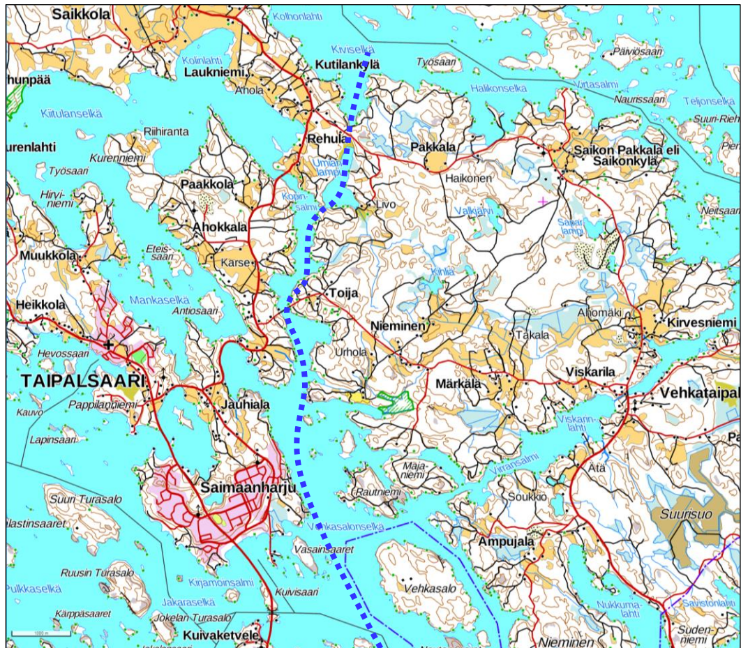
Kuva 2. Suunniteltu Kutilan kanava ja vesiväylä sijoittuvat Taipalsaaren kunnan alueelle noin 11 km pituiselle jaksolle. Varsinainen kaivettava ja ruopattava kanavaosuus sijaitsee Umianlammen ympäristössä suunnittelualueen pohjoisosassa. Suunniteltu kanava on kuvassa esitetty graafisella tarkkuudella. (ote peruskartasta, MML 2019)
