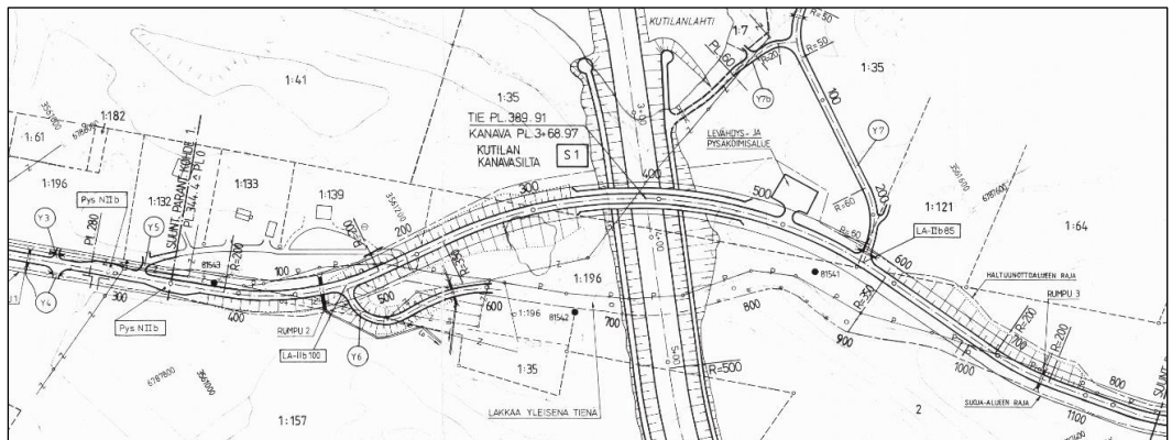
Kuva 20. Tien yleissuunnitelman vaihtoehto 1 (Tielaitos 1997).
