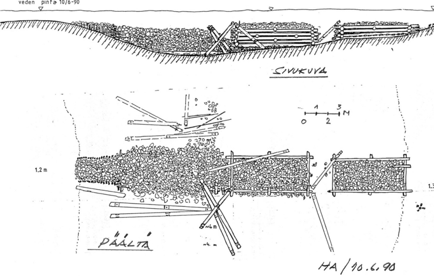
Järven pohjaan rakennettu hirsiaarkkueste Olkisalon ja Suomalansaaren välissä. Piirros Harri Heinilän työryhmä.
